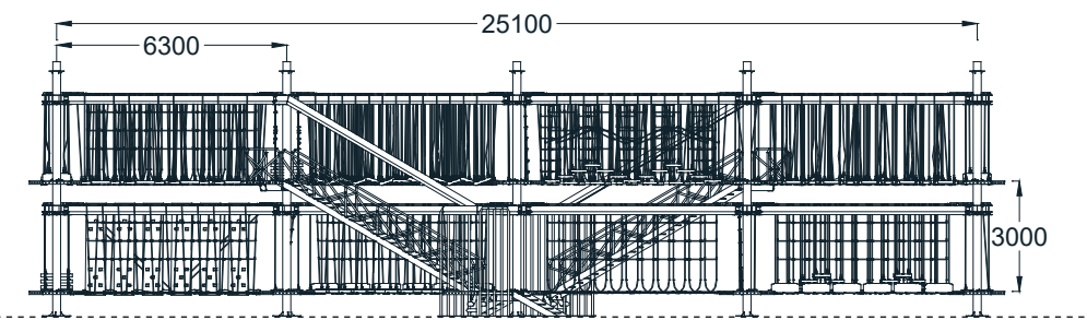
YAN GÖRÜNÜŞ / SIDE VIEW
